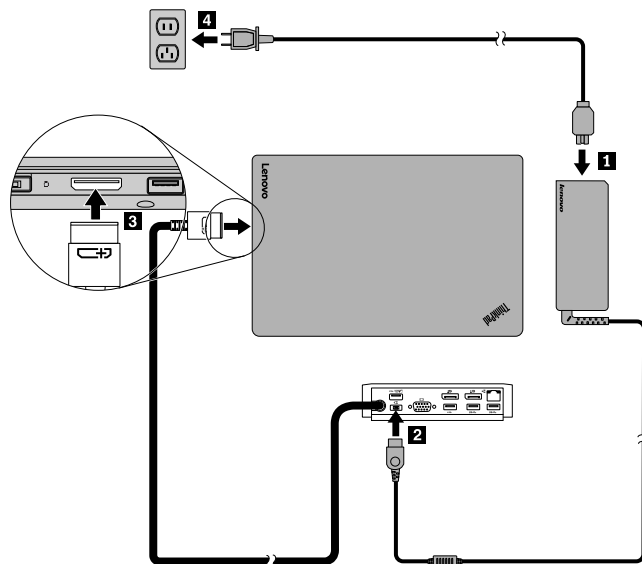
Abbildung 2. Andockstation an Netzteil und Ihren Notebook-Computer anschließen
